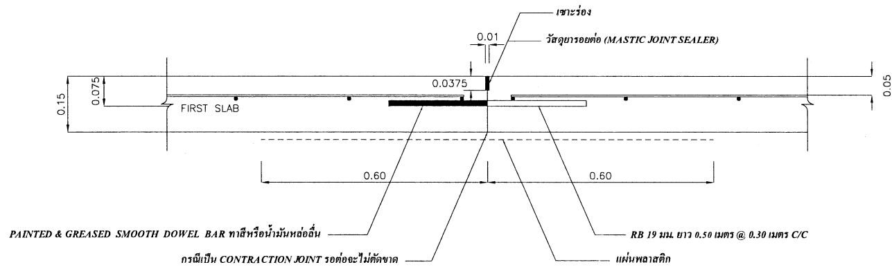
ขยายรอยต่อ CONSTRUCTION JOINT
